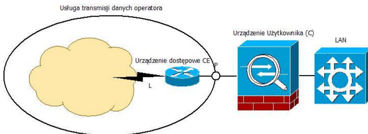
Rys.1. Architektura dostępowa.
